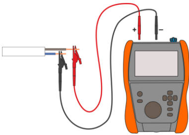
Standard R ISO -Messung
