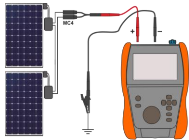
R ISO -Messung in PV-Anlagen mit Optimierern
